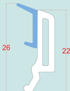
JUNQUILLO T.P 34-36MM KOM 512
