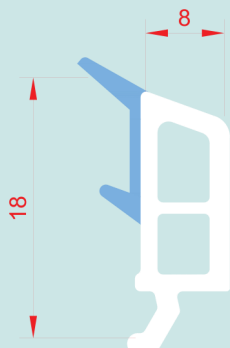
JUNQUILLO T.P 31-33 MM KOM 506
