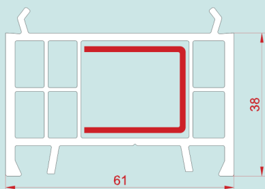
ELEVADOR MARCO 61X38MM KOM 423
