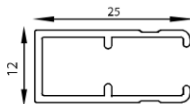
1204 Bastidor
