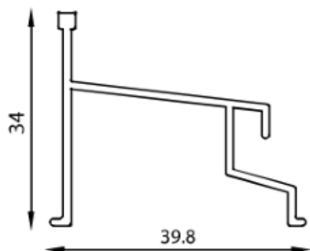
1201 Riel Inferior
