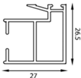
2019 Traslapo
