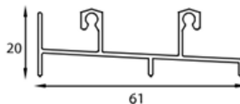
2002 Riel Inferior
