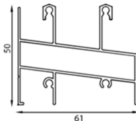
2013 Riel cámara de agua
