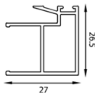
2016 Traslapo Termopanel
