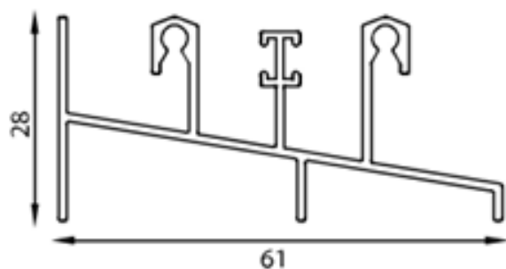
2014 Riel zona lluviosa
