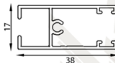
2004 Cabezal
