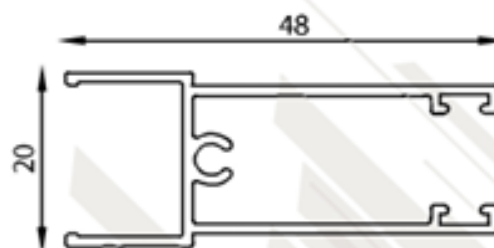
2018 Zócalo Termopanel
