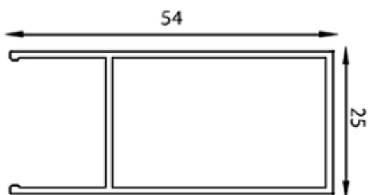
2518 Batiente T.P.
