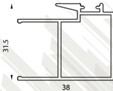
2519 Traslapo T.P.
