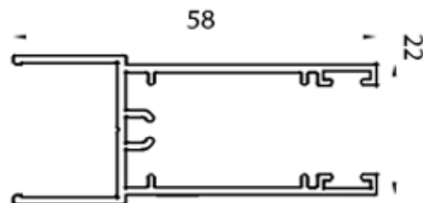
2516 Zócalo/Cabezal T.P.
