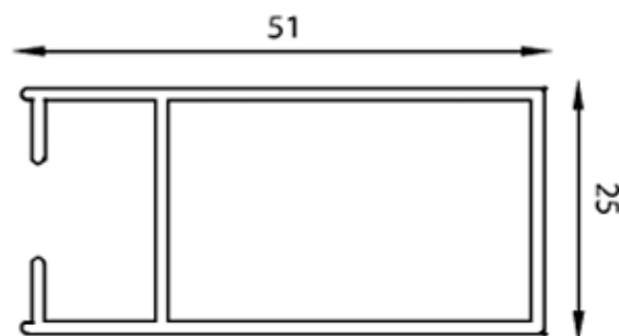
2510 Batiente
