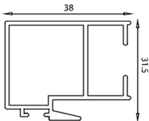
2507 Traslapo
