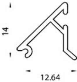
3503 Junquillo 45°
