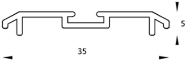
3507 Tapa portafelpa
