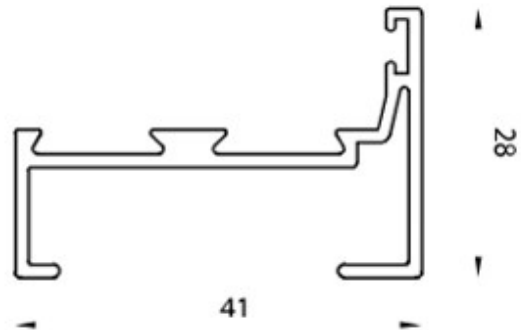
3502 Marco
