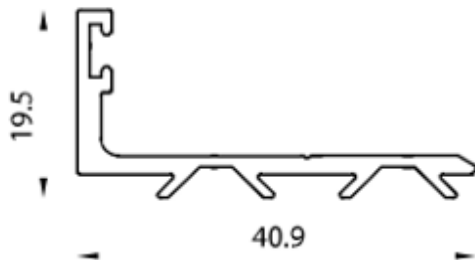
3509 Traslapo puerta
