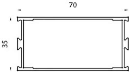
3501 Bastidor
